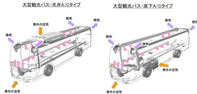
三菱ふそうエアロエースの車内空調イメージ
